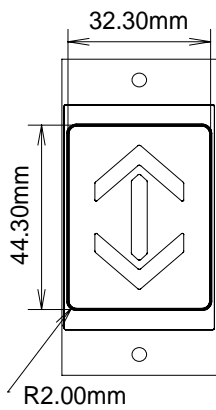
Ausschnitt Deckplatte
