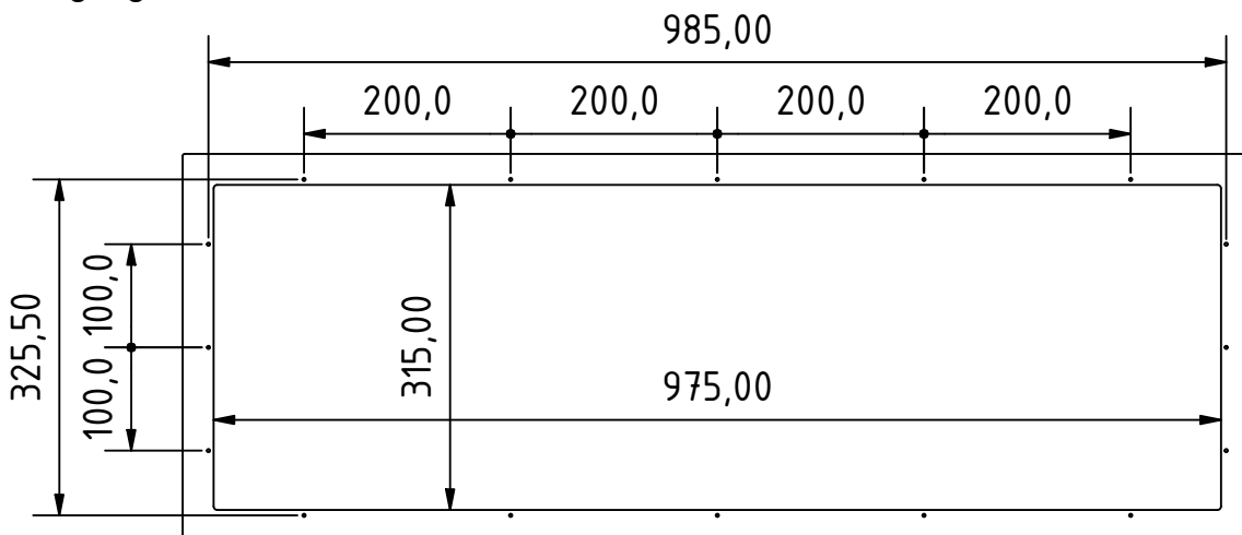
Ausschnitt im Trägerblech & Befestigungsbolzen
