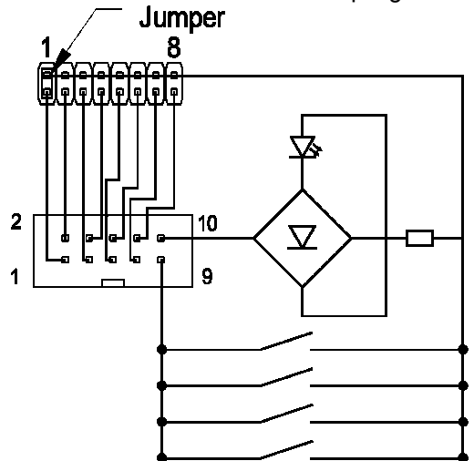
Anschluss Flachbandkabel 10 polig
