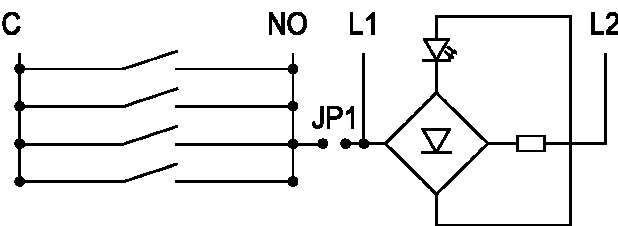
Anschluss 4 Drahttechnik, Schraubklemme
